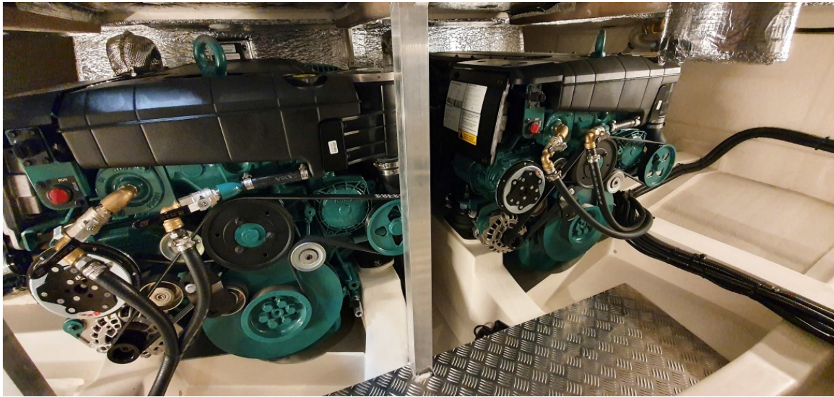
Motorraum mit 2 x Volvo Penta D 4/ 320
